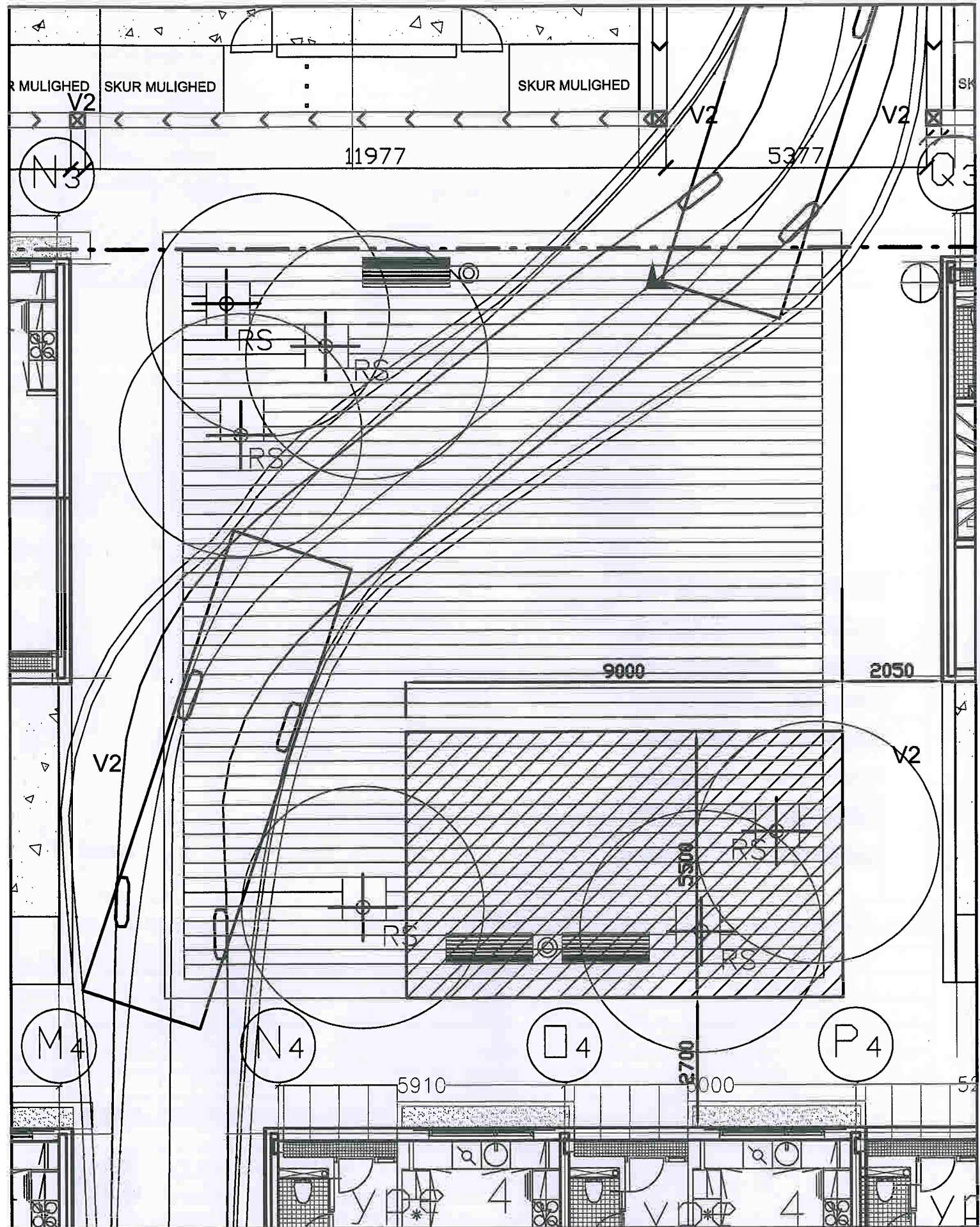
ØST TORV PLADSINDRETNINGSBEGRÆNSNINGER 1:100
